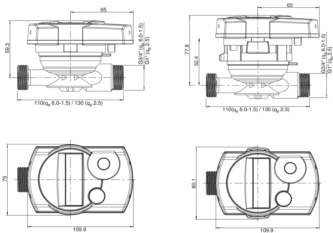
Рис.: Размеры компактных однопоточных счетчиков серии SENSOSTAR ® 2 и SENSOSTAR ® 2+ Dimensions of the single-jet compact heat meter SENSOSTAR ® 2 and SENSOSTAR ® 2+
