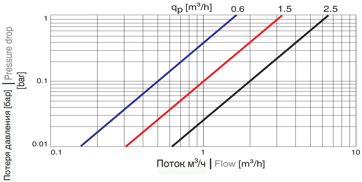
Рис.: потери давления компактного теплосчетчиков SENSOSTAR® 2 Q-Star и SENSOSTAR® 2+ Q-Star Pressure drop of the compact heat meters SENSOSTAR® 2 Q-Star and SENSOSTAR® 2+ Q-Star
