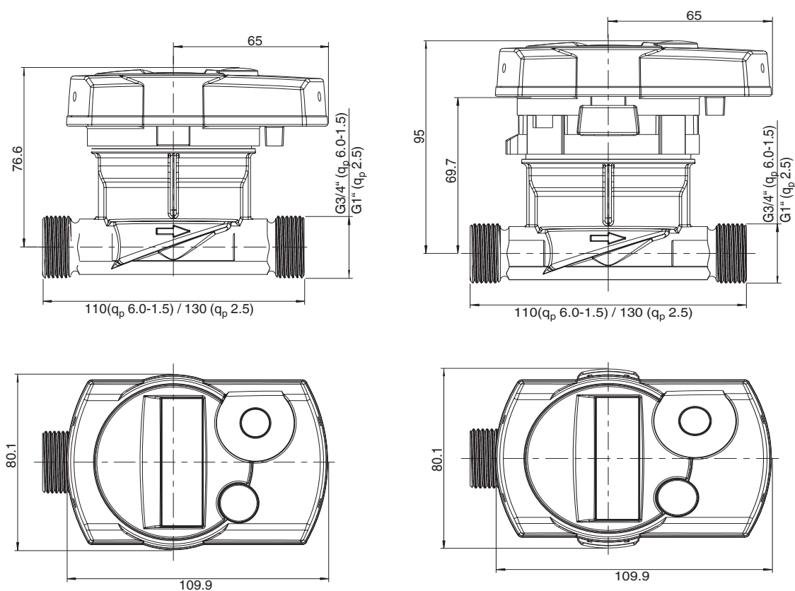
Рис.: Размеры компактных счетчиков SENSOSTAR® 2 Q-Star и SENSOSTAR® 2+ Q-Star Dimensions of the compact heat meters SENSOSTAR® 2 Q-Star and SENSOSTAR® 2+ Q-Star
