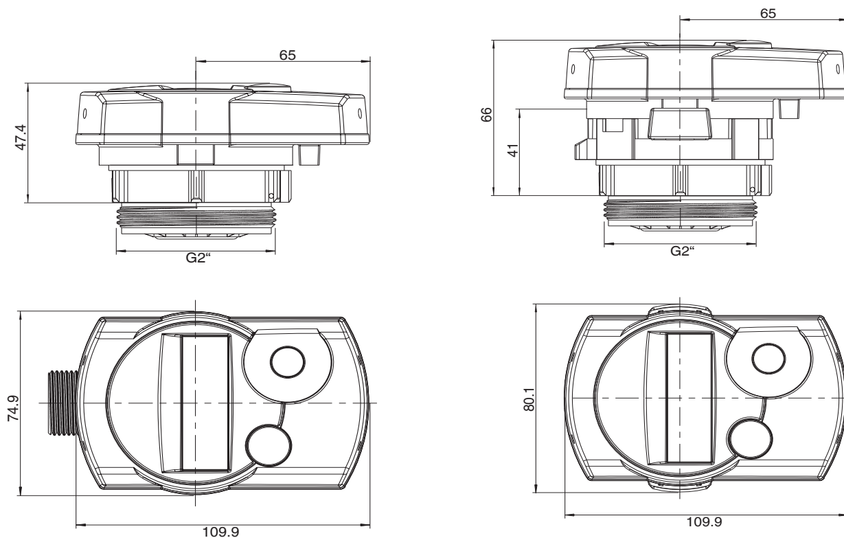
Рис: Размеры компактного многопоточного тепломера серии SENSOSTAR® 2 и SENSOSTAR® 2+ Dimensions of the coaxial multi-jet compact heat meter SENSOSTAR® 2 and SENSOSTAR® 2+
