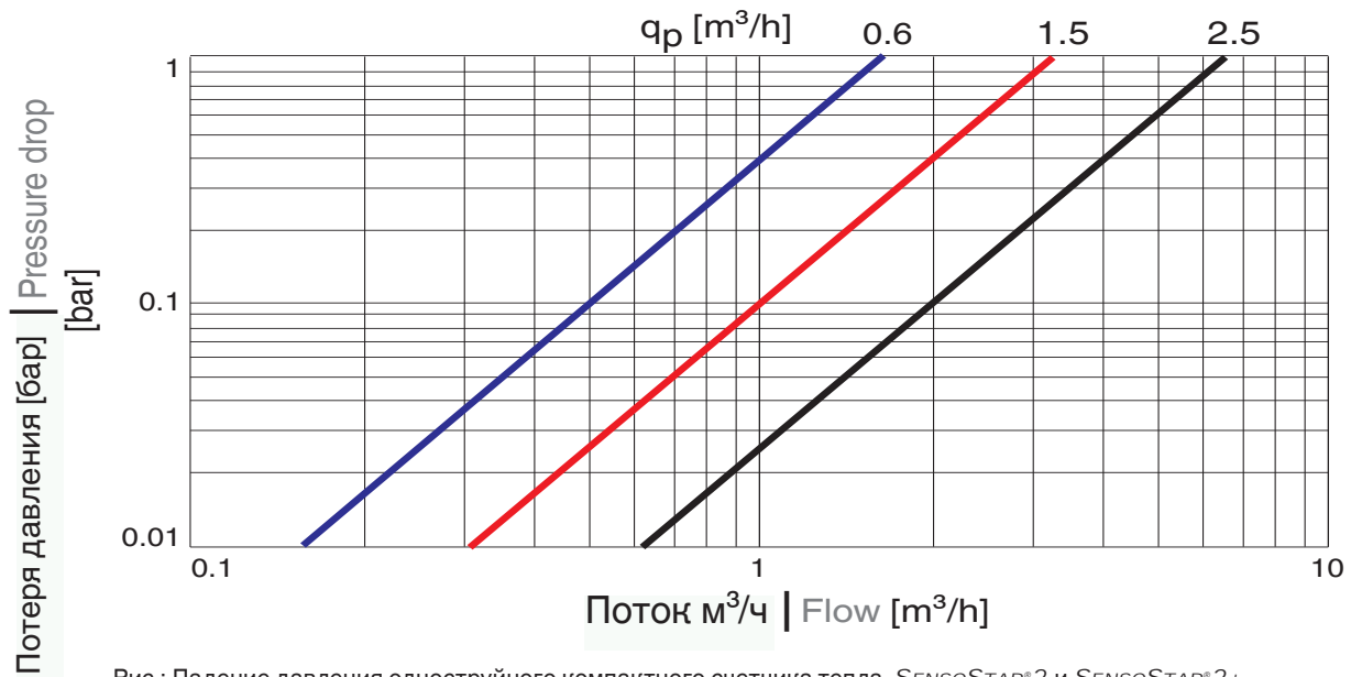
Рис.: Падение давления одноструйного компактного счетчика тепла SENSOSTAR® 2 и SENSOSTAR® 2+ Pressure drop of the single-jet compact heat meter SENSOSTAR® 2 and SENSOSTAR® 2+
