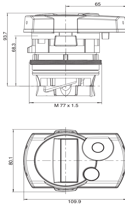
Рис.: Размеры компактного многопоточного коаксиального AStar теплосчётчика SENSOSTAR®2+ Dimensions of the AStar coaxial multi-jet compact heat meter SENSOSTAR®2+
