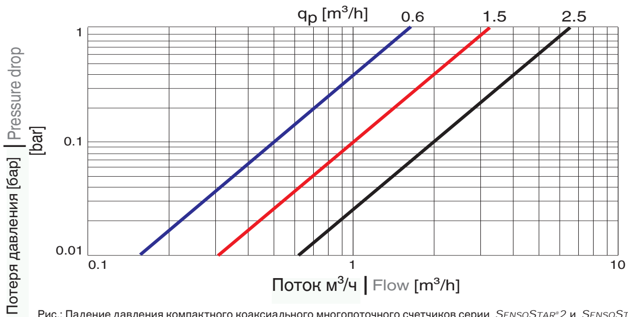
Рис.: Падение давления компактного коаксиального многопоточного счетчиков серии SENSOSTAR® 2 и SENSOSTAR® 2+ Pressure drop of the coaxial multi-jet compact heat meter SENSOSTAR® 2 and SENSOSTAR® 2+
