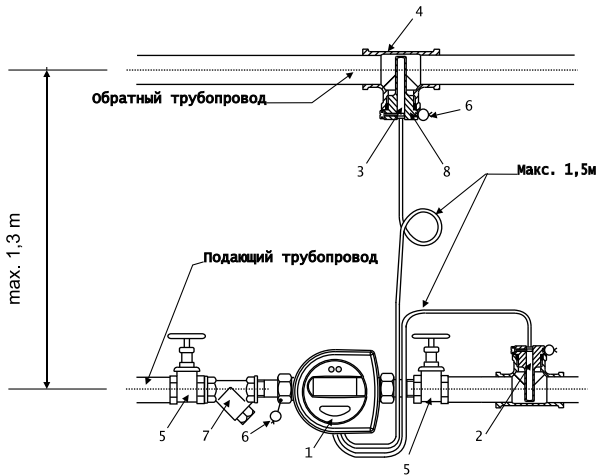
Рис. 4 Монтаж счетчика тепла в горизонтальный трубопровод. Счетчик тепла повернут на 90°С
