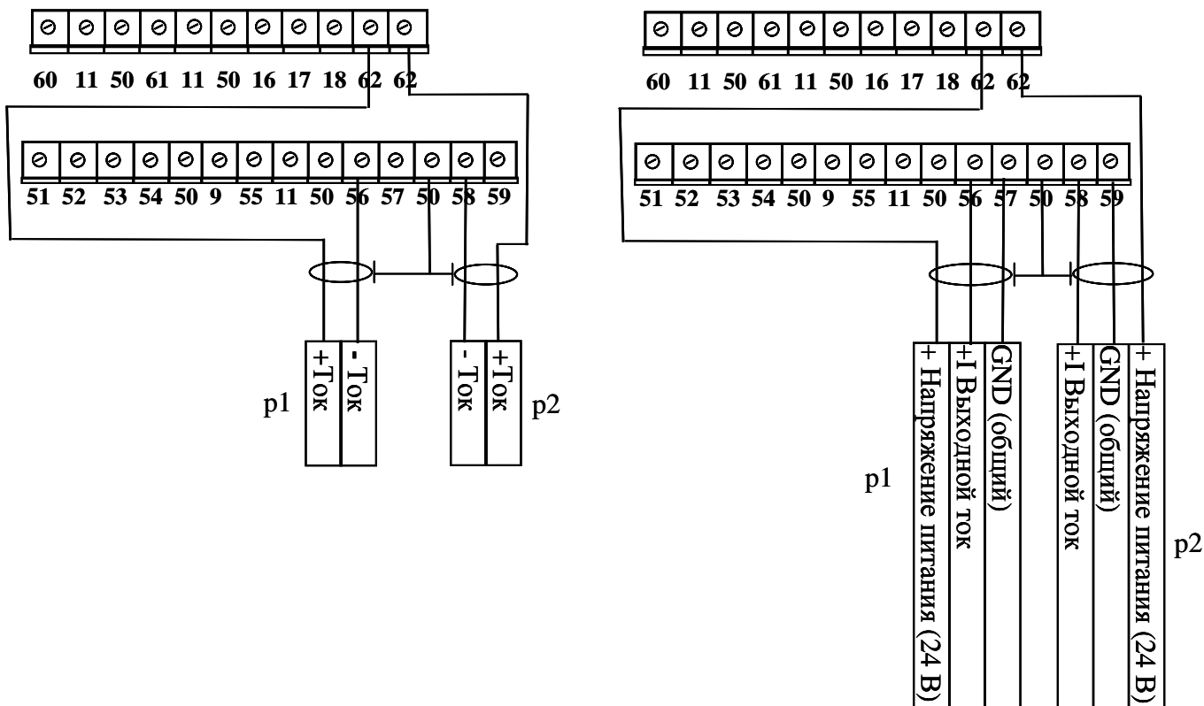
а) Двухпроводная схема подключения датчиков давления (4-20 mA), питание от вычислителя (+ 24 V)
