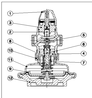
Рис.4. Устройство регулятора AVQ (P v 16)
