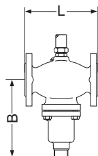
VFQ 2 DN 15 - 125
