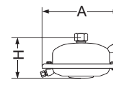
AFQ (9 kg)
