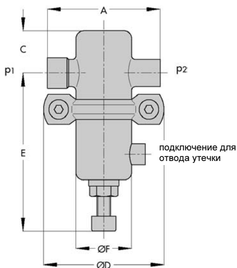
Рис. 5.3 • Серия Kvs=0,15 диапазоны заданного давления 0,3...20 бар
