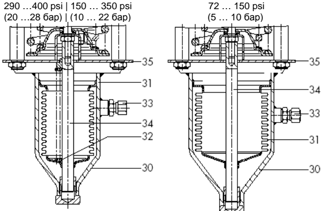
Привод с металлическим сиффоном
