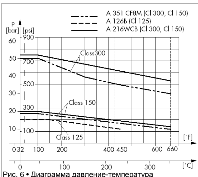
Рис. 6 • Диаграмма давление-температура
