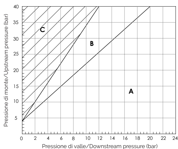
A - Campo di funzionamento raccomandato / Recommended working conditions B - Cavitazione incipiente / Incipient cavitation C - Cavitazione dannosa / Dangerous cavitation
