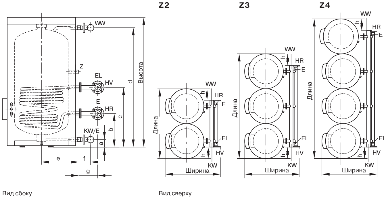
Вид сбоку
