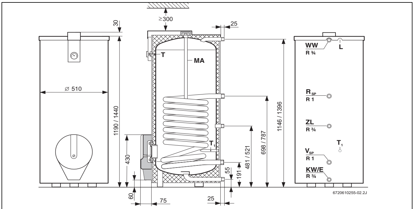
Рис. 3 Розміри за косяю рискою стосується більшої конструкції бойлера.
