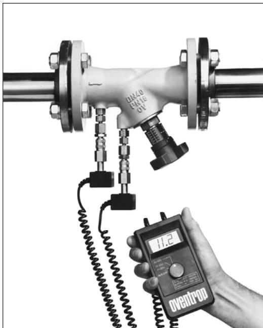
Elektronisches Differenzdruckmessgerät, Artikel-Nr. 106 91 52
