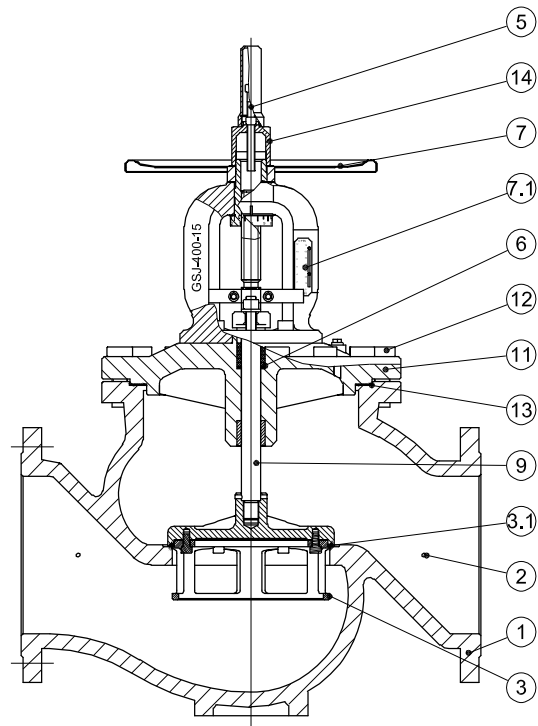
MSV-F2 DN 200 - 300
