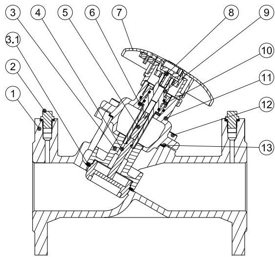
MSV-F2 DN 65
