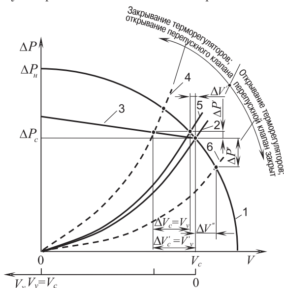
Рис. 6.43. Работа перепускного клапана:
