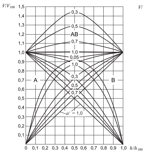
Рис. 6.22. Линейная/линейная рабочая расходная характеристика трехходового клапана
