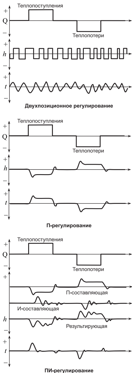
Рис. 6.56. Регулирование температуры воздуха калорифером системы воздушного отопления
