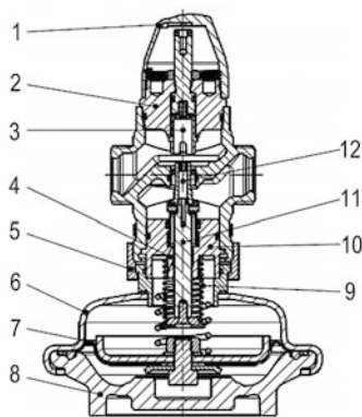
Рис. 6.34. Устройство регулятора расхода AVQ:
