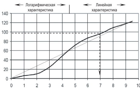
Рис. 6.15. Расходная характеристика клапана MSV-F2 d_y = 80 мм
