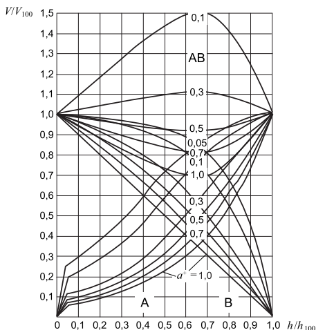
Рис. 6.24. Логарифмическая/линейная рабочая расходная характеристика трехходового клапана
