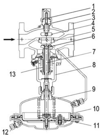
Рис. 6.31. Устройство регулятора перепада давления AFPB-F/VFQ
