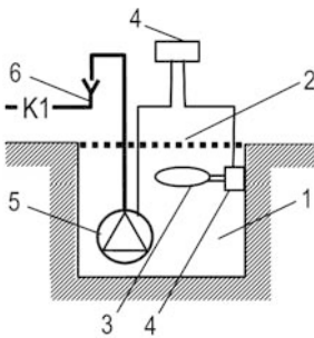
Рис. 2.17. Отвод воды в тепловом пункте: 1 – приямок; 2 – решетка; 3 – датчик уровня; 4 – контроллер; 5 – дренажный насос; 6 – трубопровод бытовой канализации
