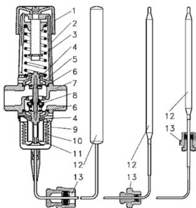
Рис. 6.37. Устройство регулятора температуры AVTB:
