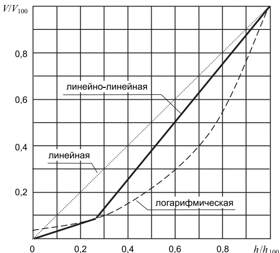
Рис. 6.17. Линейно-линейная идеальная расходная характеристика клапана
